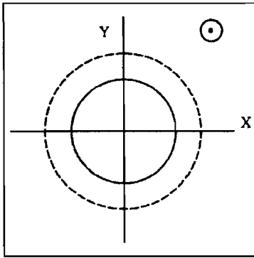
G- الحالة الأولى لاستقطاب الموجة التجاذبية
